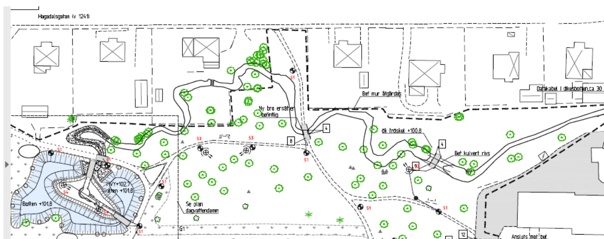
Bild 2: Visar översiktsritning över Hagadalsparken, med dagvattendamm och stigar samt broar.
